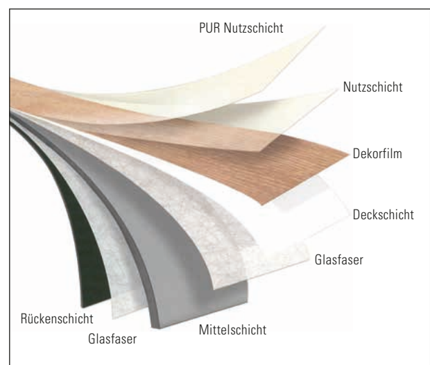
Schichtaufbau eines Designbelags, Foto: Moduleo
